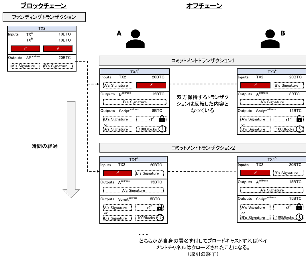
図表 57 ペイメントチャネルの更新の意味
