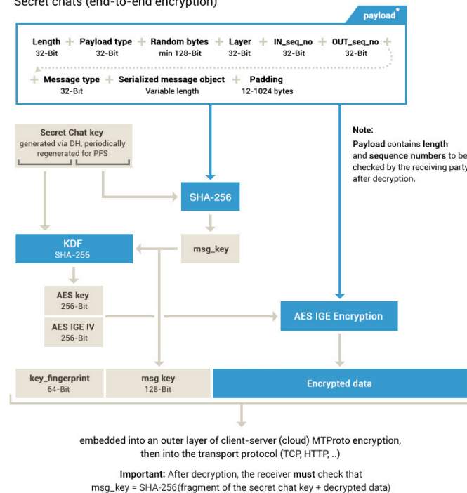
図表 113 Telegram の暗号化プロトコル MTPROTO 308
