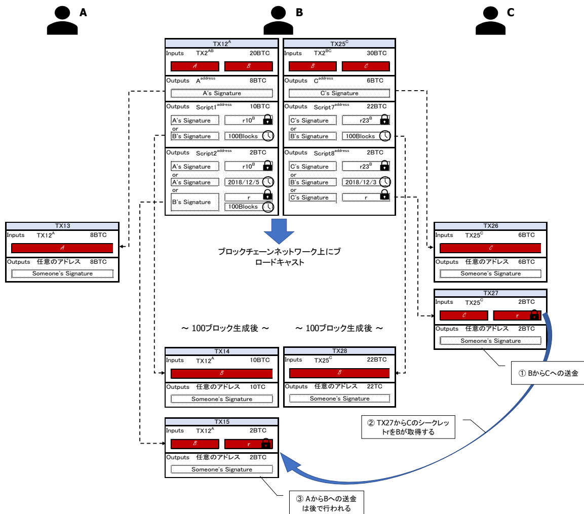
図表 62 複数のペイメントチャネルのクローズと A から C への送金
