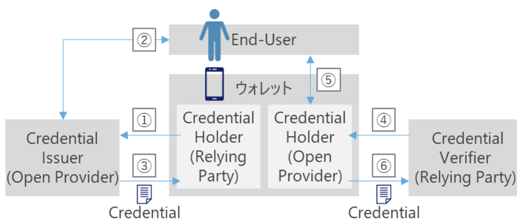
図 0-17 : OpenID Connect Claims Aggregation の過程
