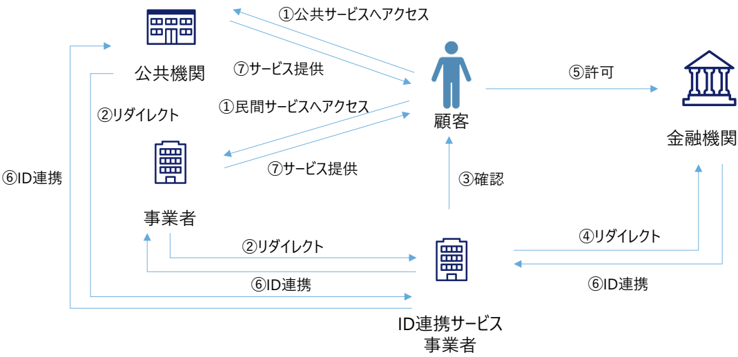
図 2- 48 金融機関が作成したデジタルアイデンティティを用いた ID 連携フロー
