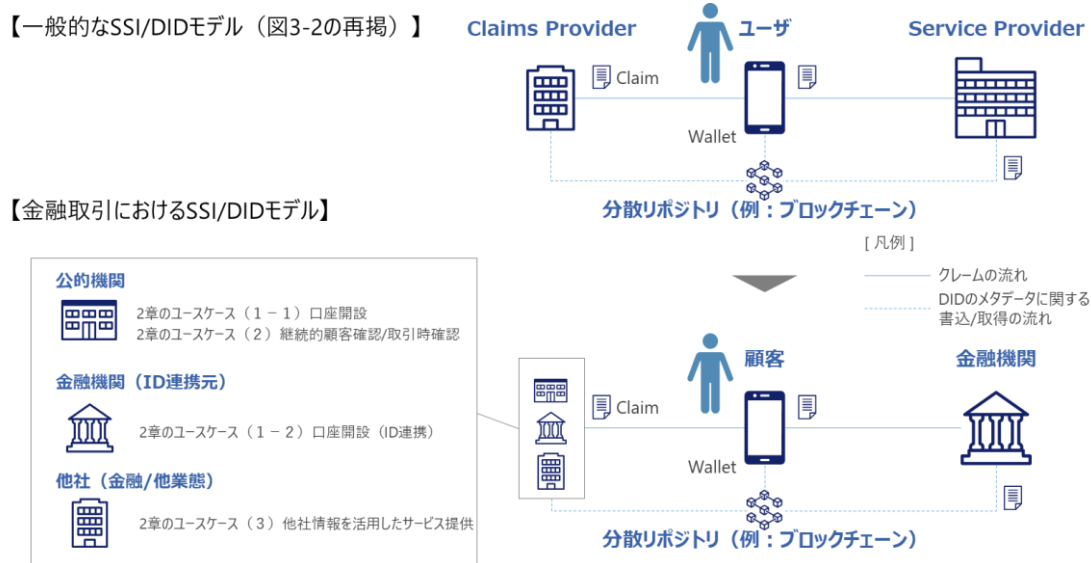
図 0-67：金融取引における SSI/DID モデル
