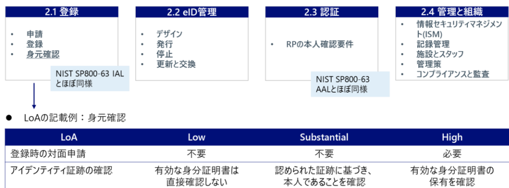
図 2-18 (参考) 米国・EU のアイデンティティ保証フレームワーク
