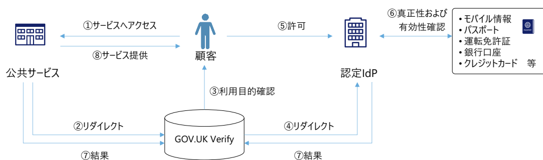
図 2- 38 GOV.UK Verify における本人確認フロー 149
