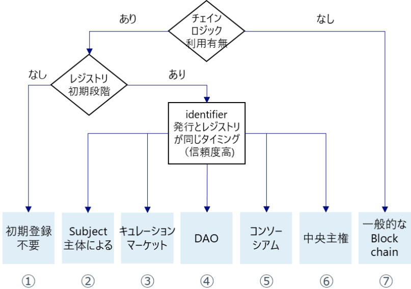
図 0-55 : Identifier のレジストリモデル 253
