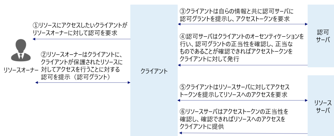
図 1-14 : OAuth 2.0 の概観の流れ 64
