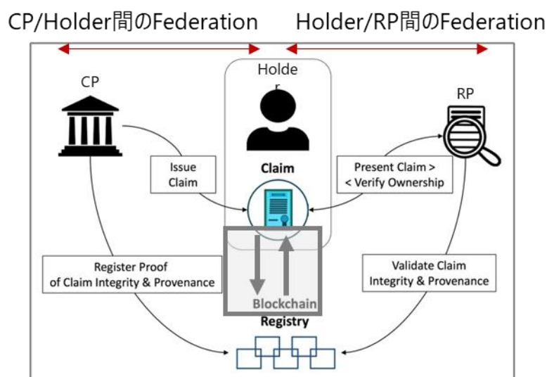
図 0-83：ローカルに ID プロバイダ機能をデプロイする場合の SSI モデル実現像 283
