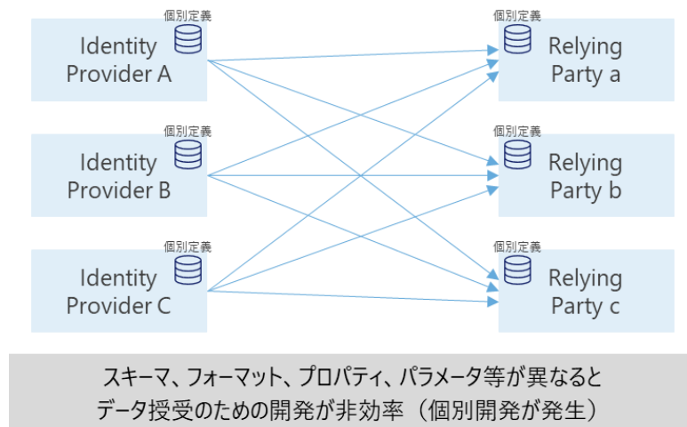
図 0-56：個別フォーマット・スキーマ等が定義された状態でのデータ連携
