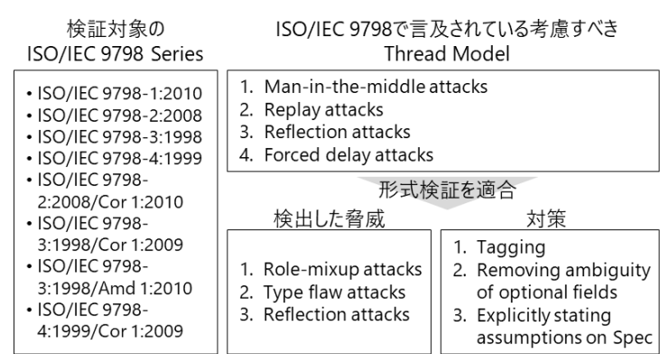
図 0-64 : ISO/IEC 9798 に対する形式検証適合と検出脅威例
