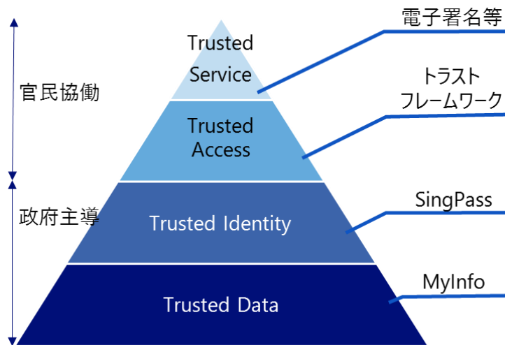
図 2- 35 NDI Stack の概要 140
