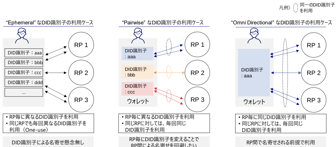
図 0-79 : DID 識別子の使い方
