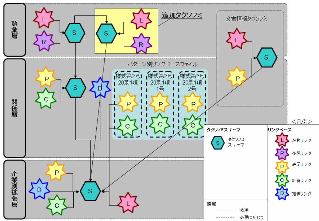
図 1 追加タクソノミのアーキテクチャ (案)
